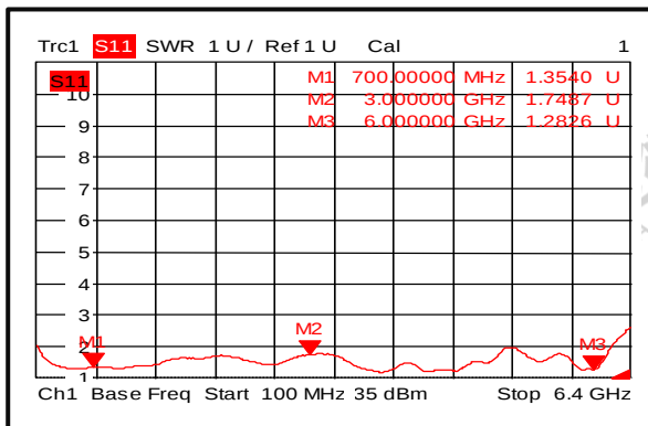
输入驻波比 (-45℃)
