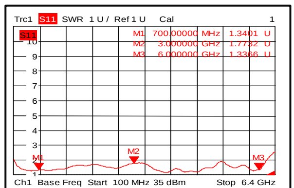
输入驻波比 (+85℃)
