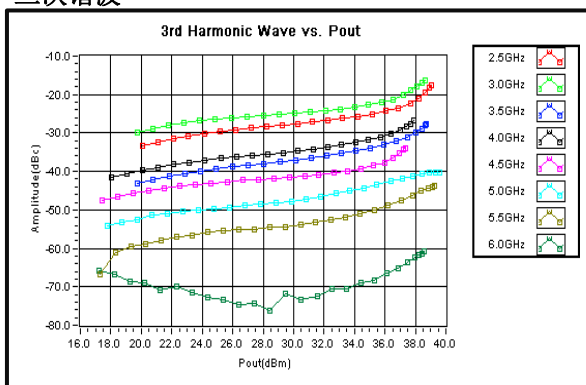
三次谐波
