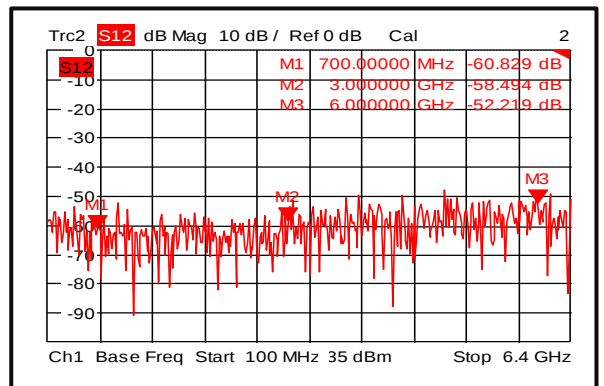
隔离度 (-45℃)
