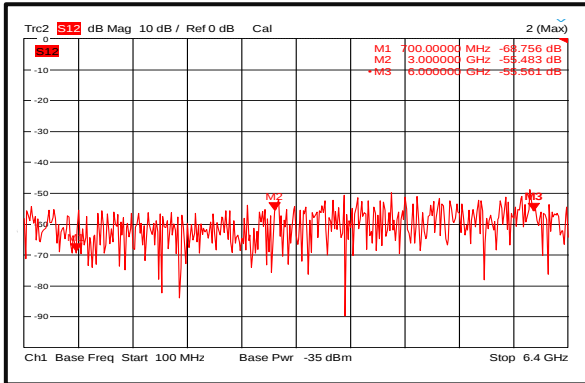
隔离度 (+25℃)
