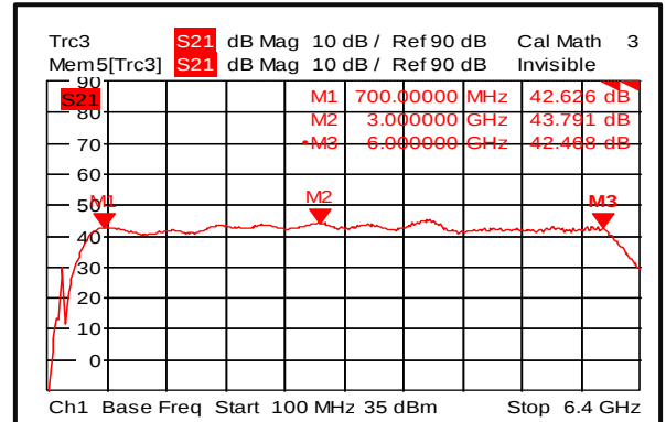
增益 (-45℃)
