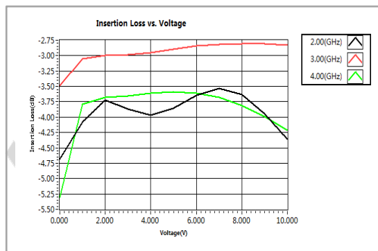
插损/电压
