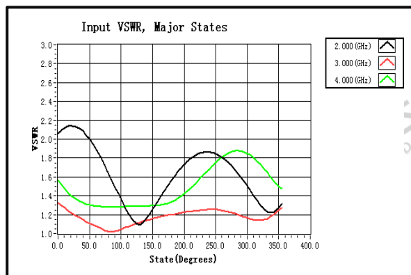
输入驻波比/频率
