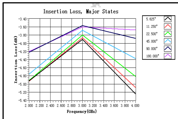
插损值/频率
