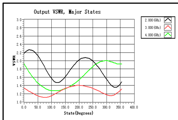
输出驻波比/频率
