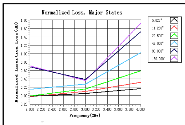
移相状态/插损
