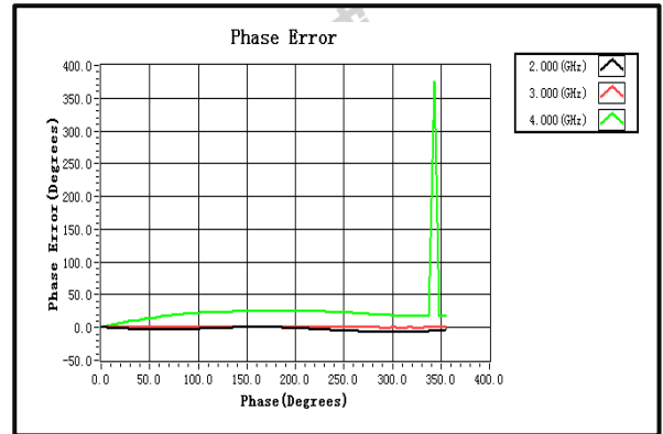
相位偏差
