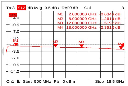
损耗 (+85℃)
