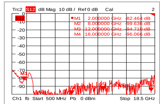
隔离度 (+85℃)
