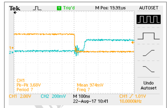
开关速度
