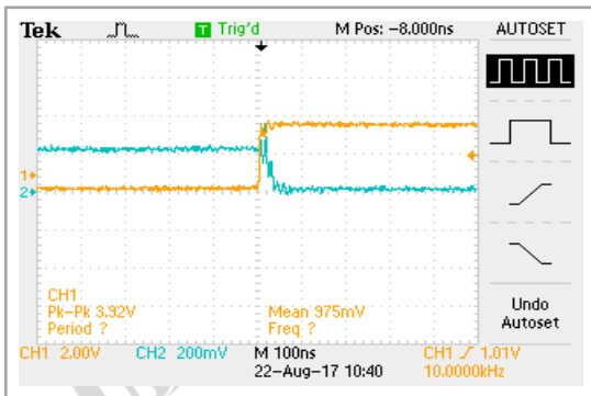
开关速度
