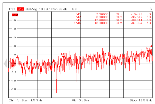
隔离度 (+25°C)
