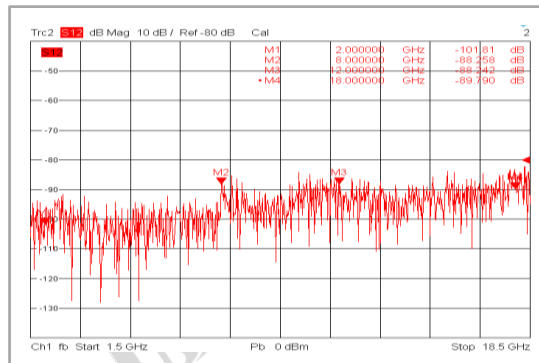
隔离度 (-45°C)
