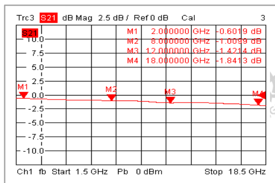
损耗 (-45°C)
