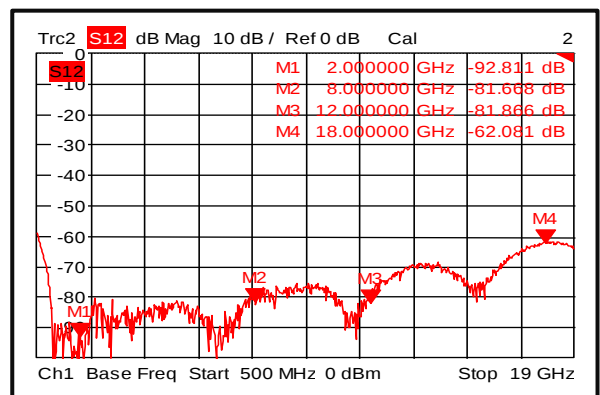
隔离度 (-45℃)
