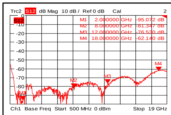
隔离度 (+85℃)
