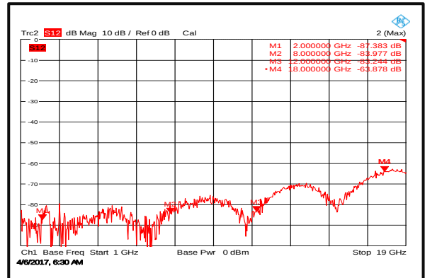
隔离度 (+25℃)
