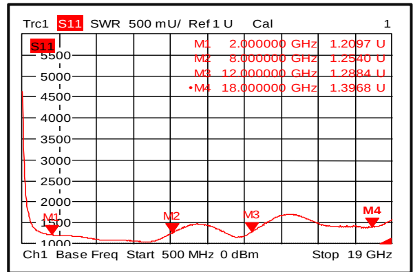
输入驻波比 (-45℃)
