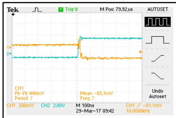
开关速度
