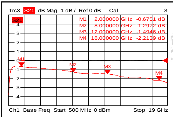
损耗 (-45℃)
