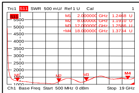
输入驻波比 (+85℃)
