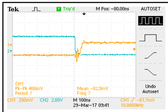
开关速度
