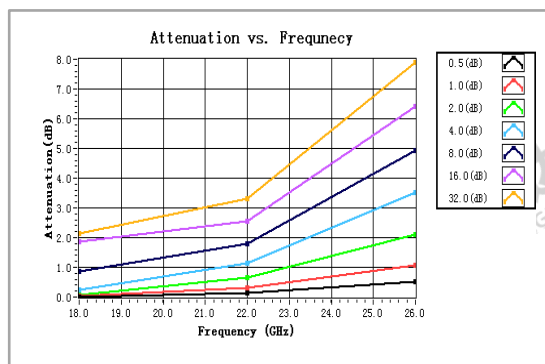
衰减值/频率
