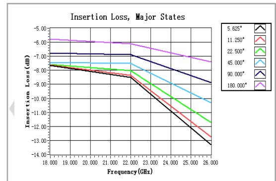
插损值/频率
