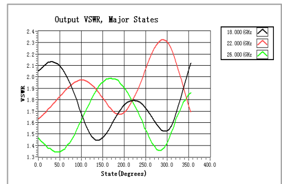
输出驻波比
