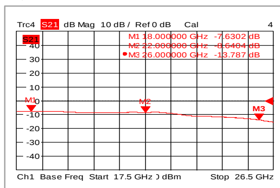
损耗（+25°C）
