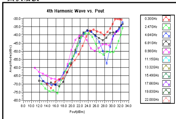
四次谐波
