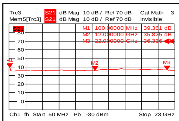
增益 (-45℃)
