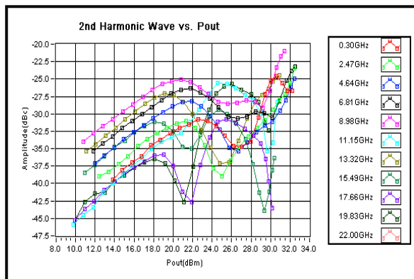
二次谐波
