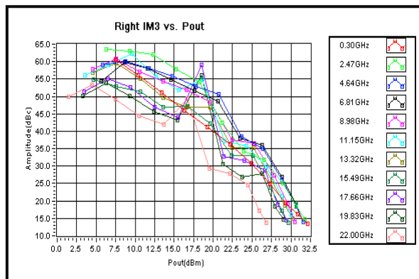
右侧IM3
