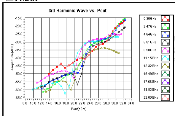
三次谐波
