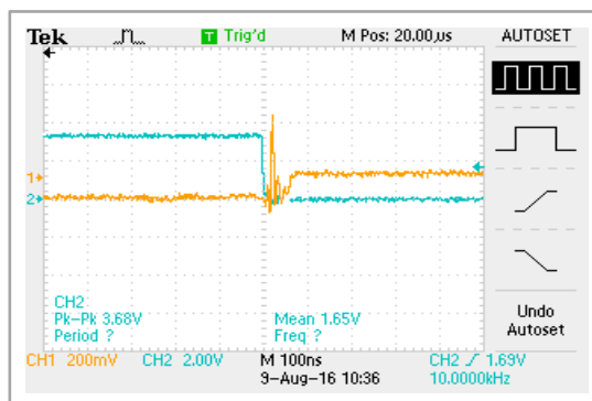
开关速度
