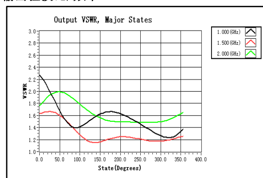
输出驻波比/频率
