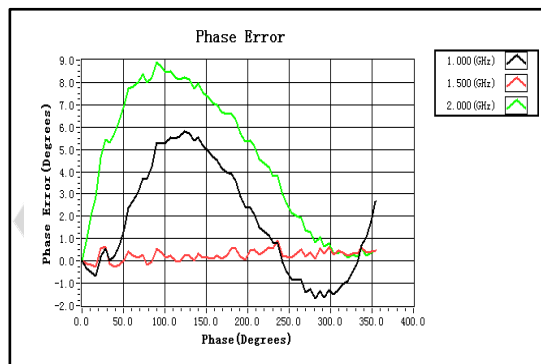
相位偏差
