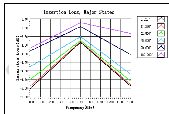
插损值/频率
