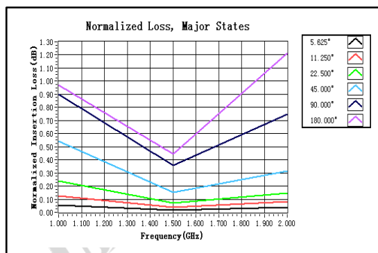
移相状态/插损
