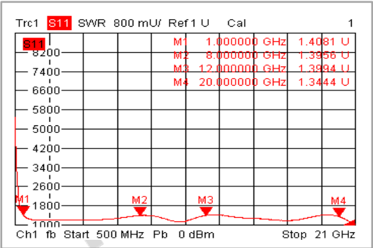
输入驻波比（+25℃）
