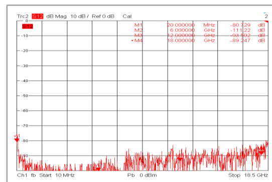
隔离度 (+85℃)
