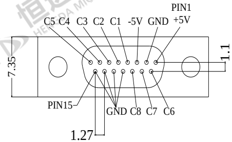
MICRO-D15 (Female)
