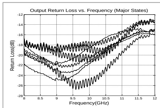
输出回波损耗/频率
