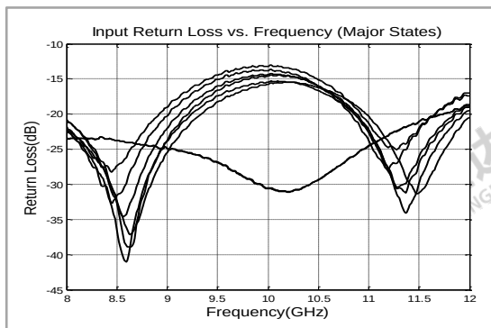
输入回波损耗/频率
