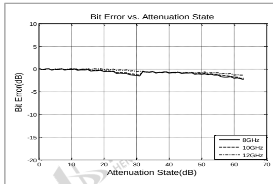
衰减步进误差
