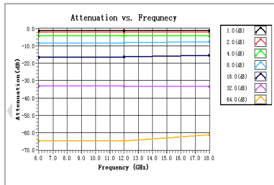
衰减/频率
