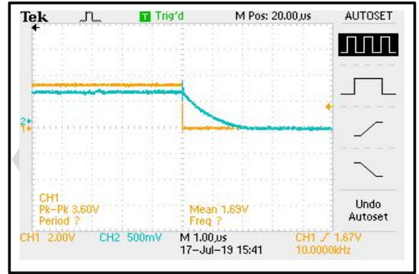
下降时间
