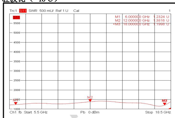
驻波比 (-45°C)
