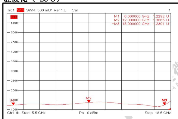
驻波比 (+25°C)
