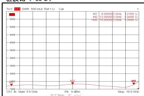
驻波比 (+85°C)
