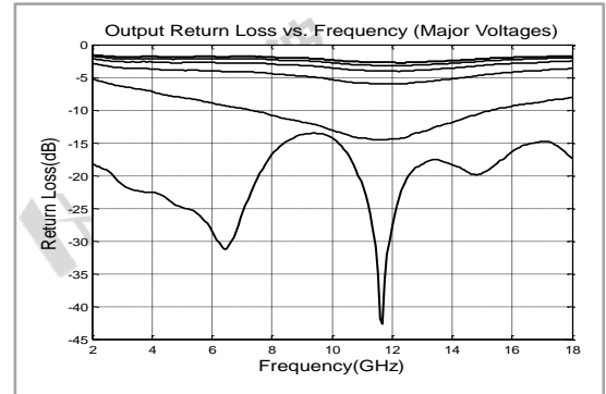
输出回波损耗/频率
