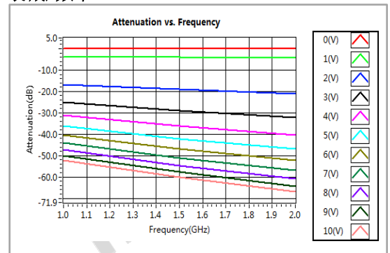
衰减/频率
