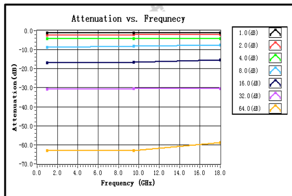
衰减值/频率
