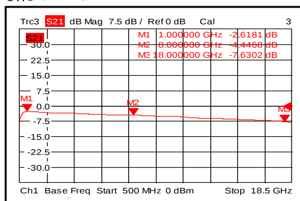
损耗 (+85℃)
