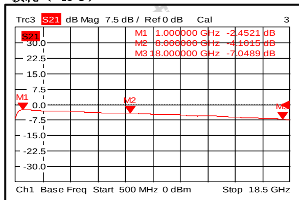
损耗 (-45℃)
