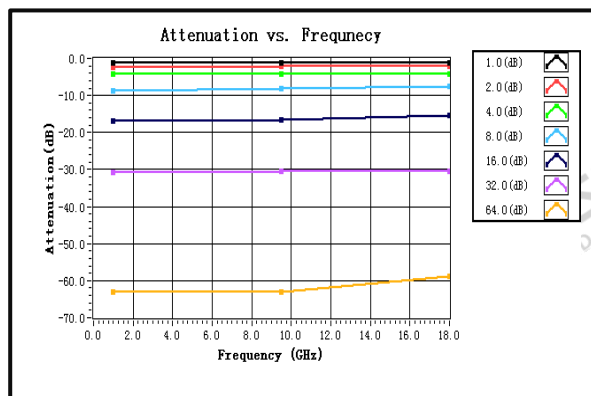
衰减平坦度/频率
